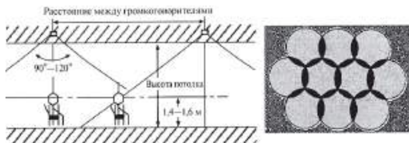
Рис. 5.8. Схема расстановки громкоговорителей
